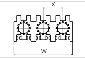
uni RTB M1 | uni RTB M2
